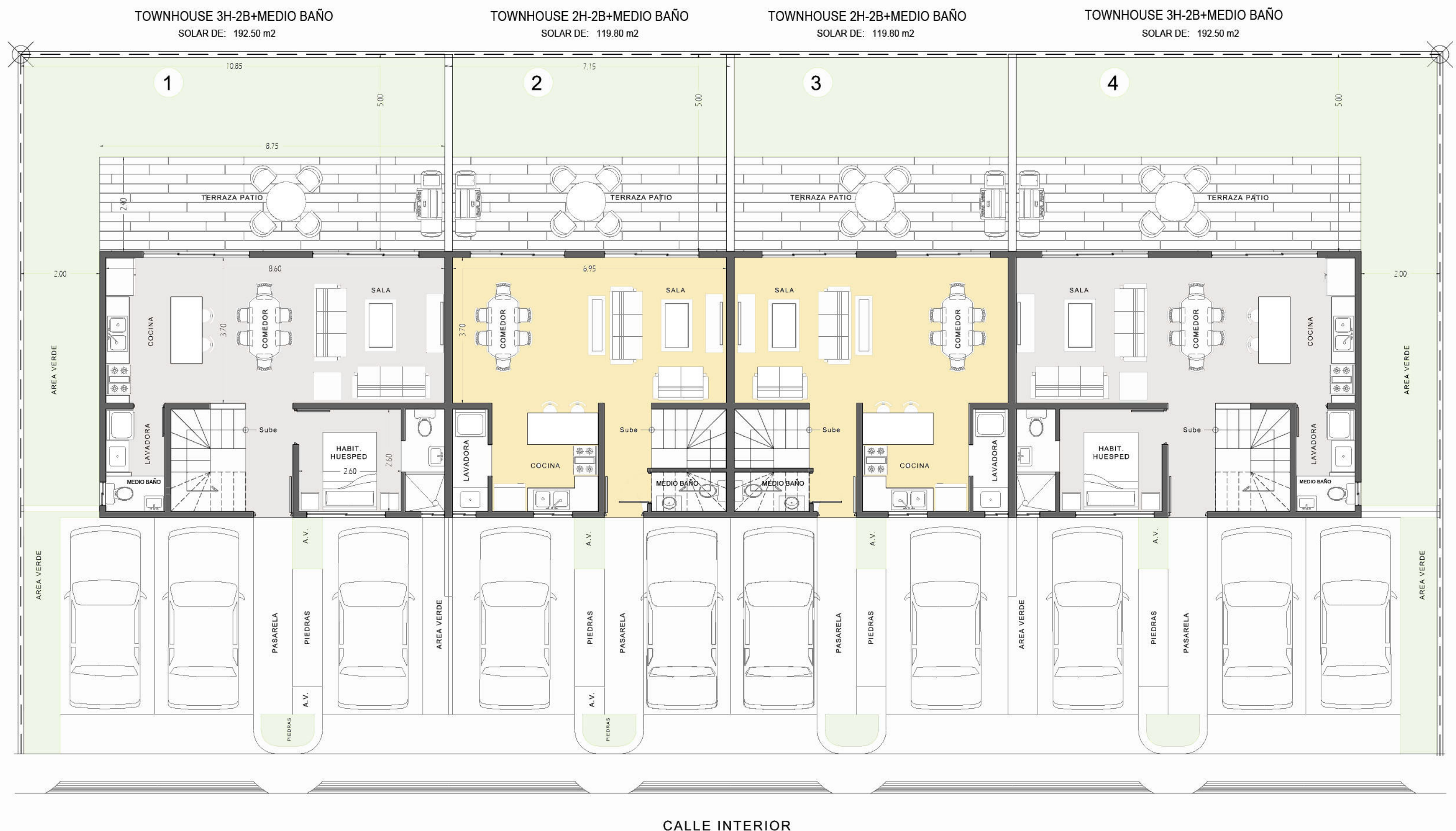
PLANTA ARQUITECTONICA AMUEBLADA 1ER NIVEL
